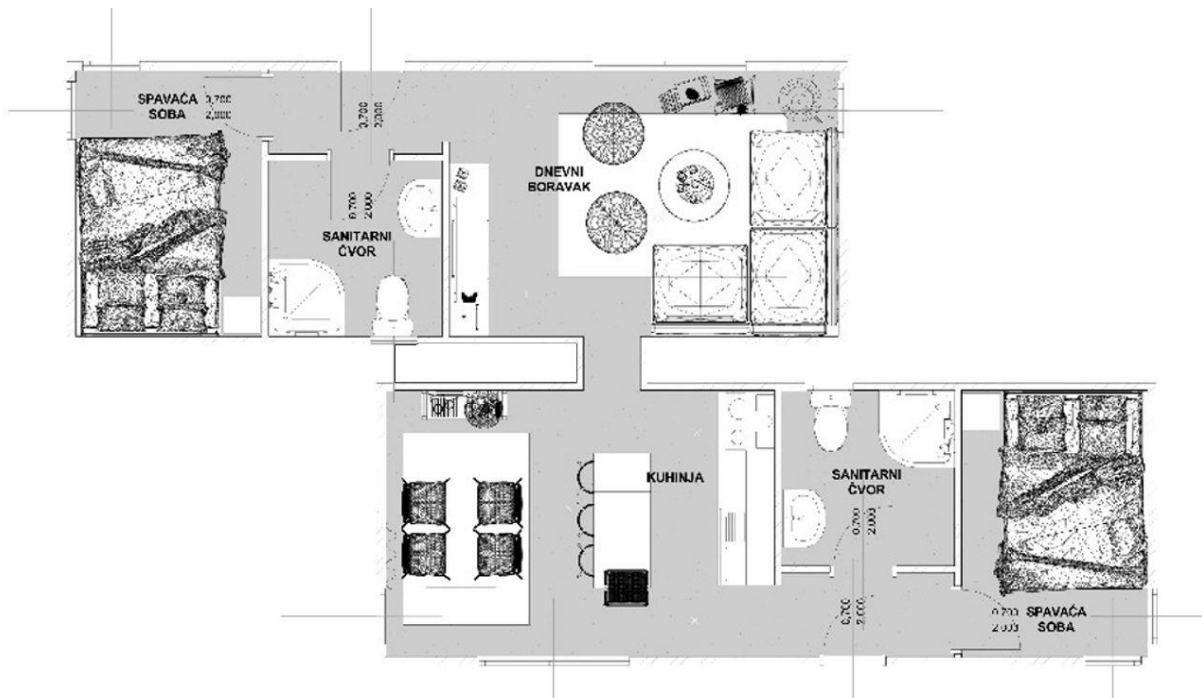
Tlocrt mobilne kuće Leona 48 L-Z
