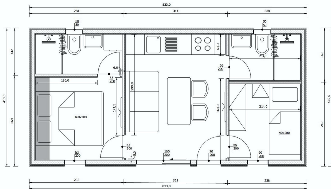
Tlocrt mobilne kuće Leona 35
